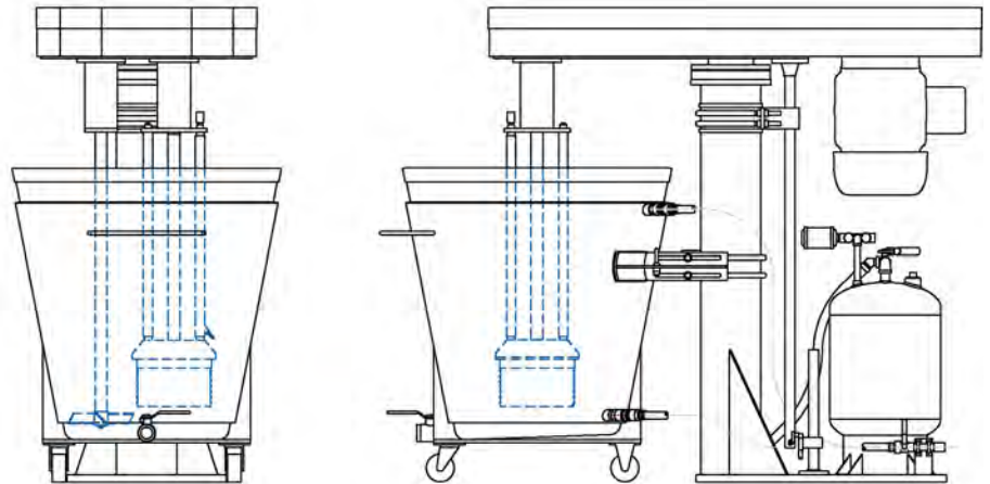
Desenho dimensional com tanque Veja tabela para dimensões
